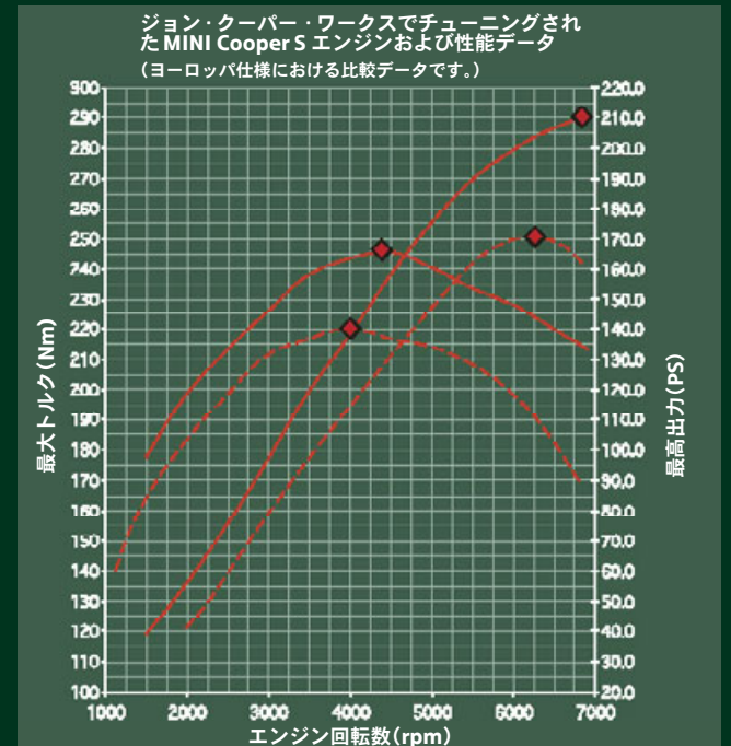
実線: チューニング・キット装着のMINI Cooper S 点線: 標準MINI Cooper S
