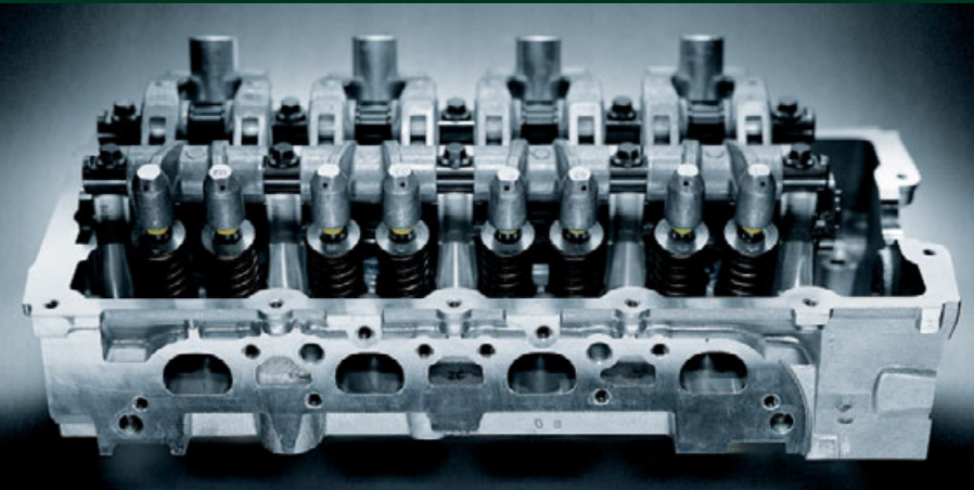
数々の開発の成果が注ぎ込まれたシリンダー・ヘッド
